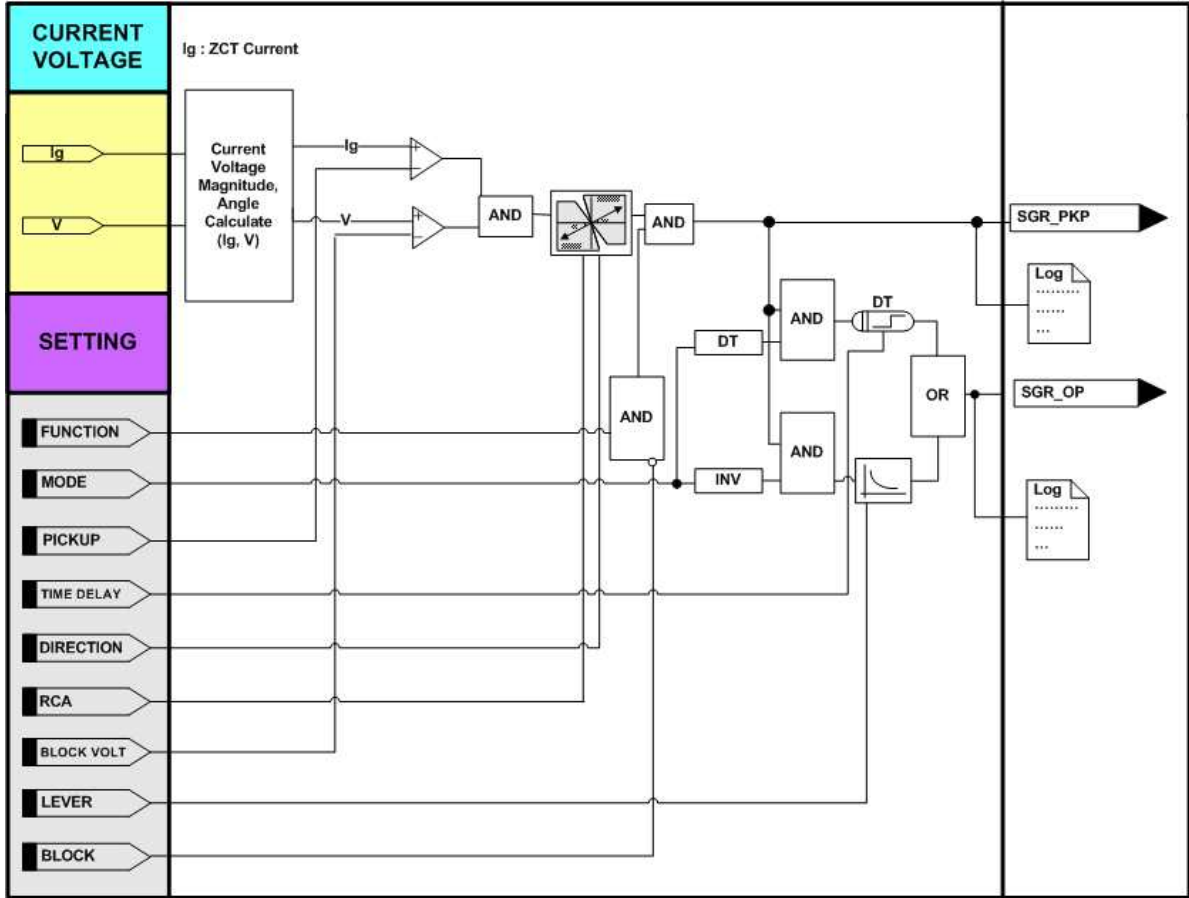
<Figure. 선택 지락과전류 (SGR) 보호 Logic Diagram>
