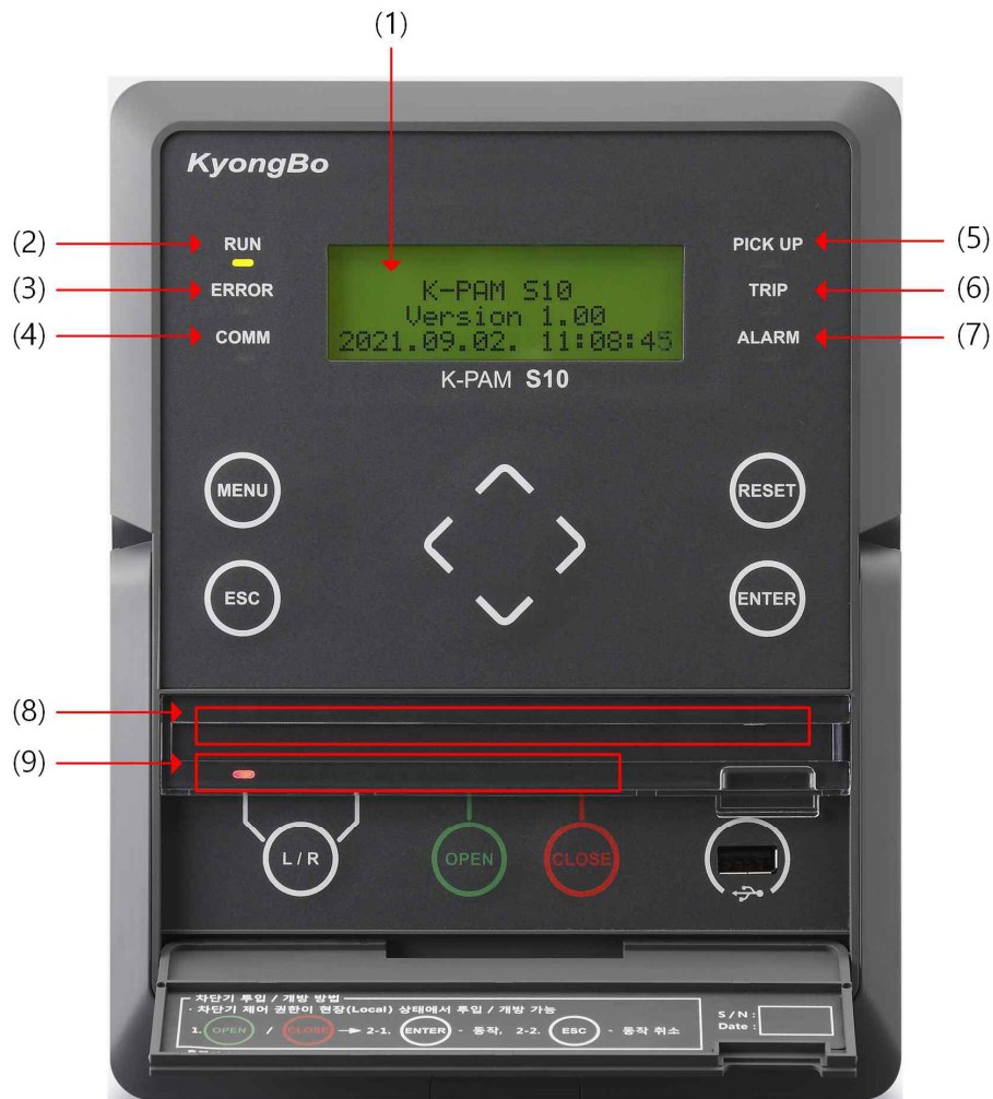
<Figure. 계전기 전면 표시조작부 구성>
