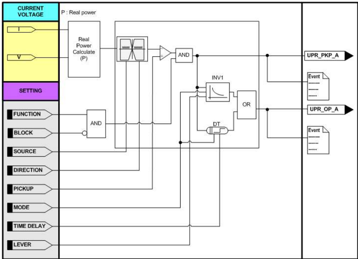
<Figure. 저전력 (UPR) 1 ~ 2 동작특성>
